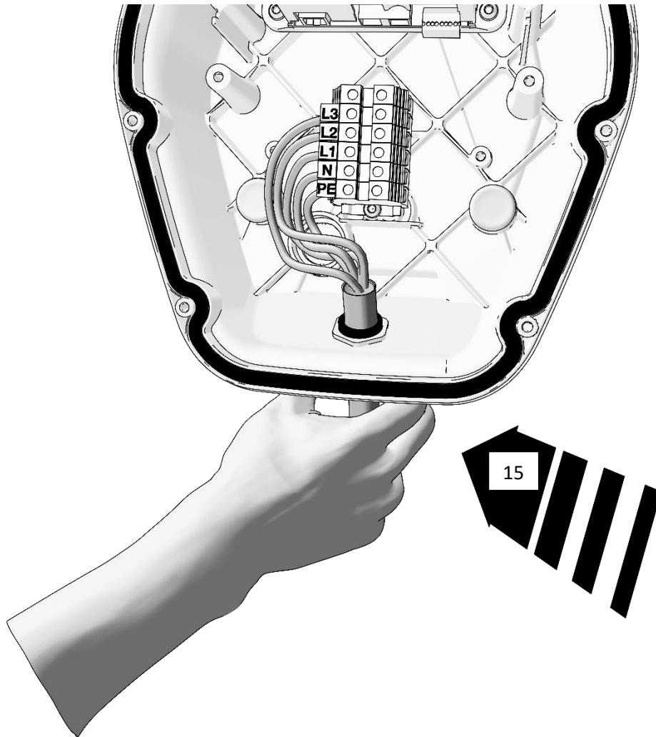
Bild 16 Kontrollieren der Kabelverschraubungen
