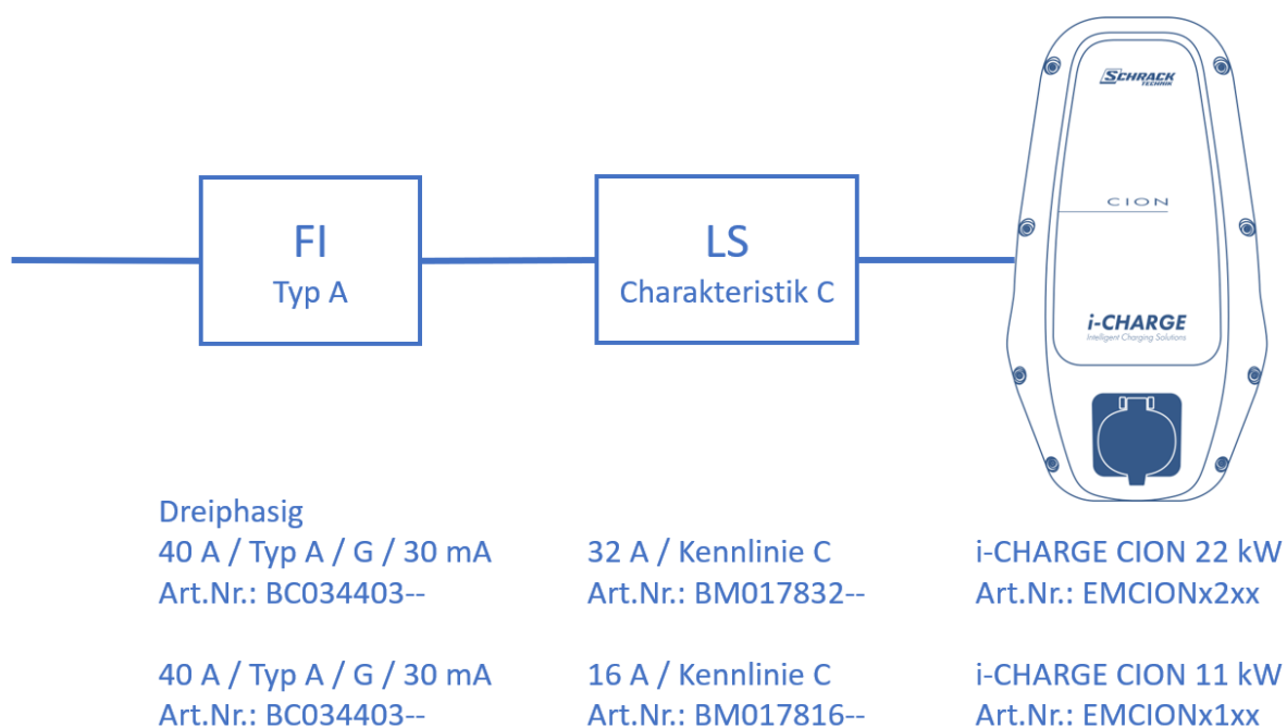
Bild 38 Vorsicherung Schema FI + LS
